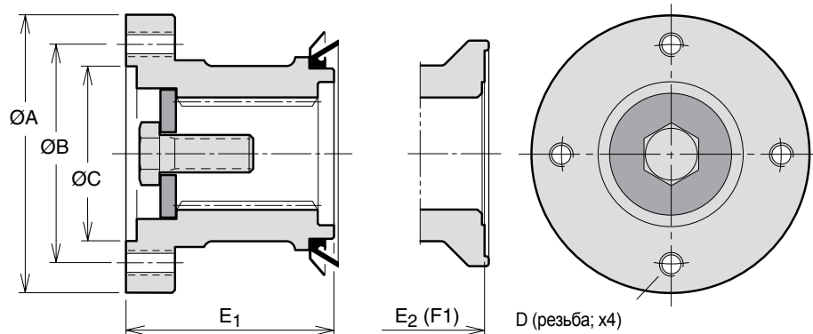
Рис. 1. DIN 90 (370 4634)
