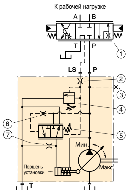
Гидравлическая схема для VP1-095/110/130
