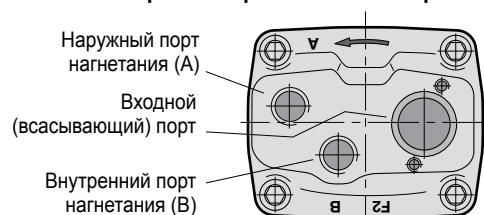
Торцевая крышка насоса с вращением по часовой стрелке
