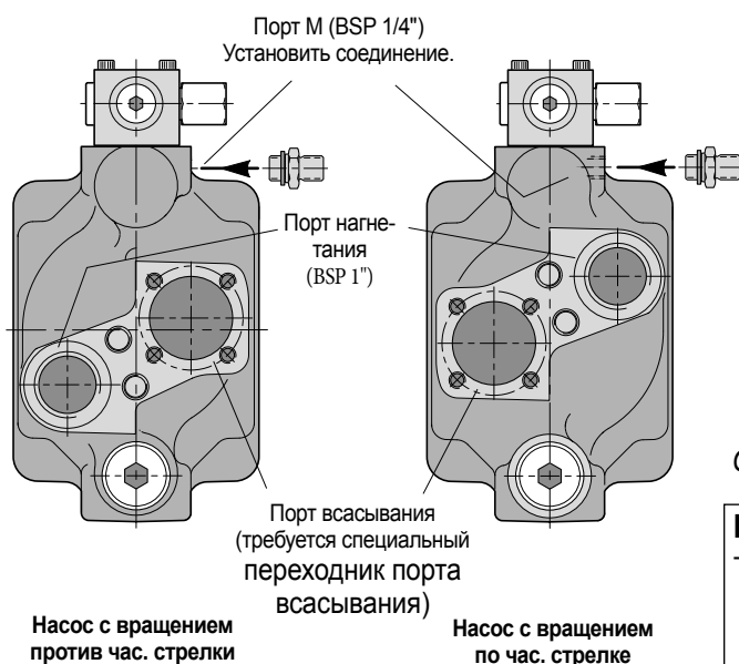
Главные порты VP1-095/-110/130 (с монтажом соединений).
