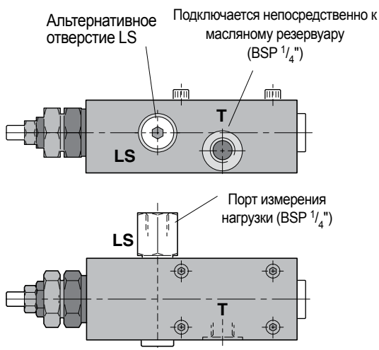
Порты регулятора с измерением нагрузки.
