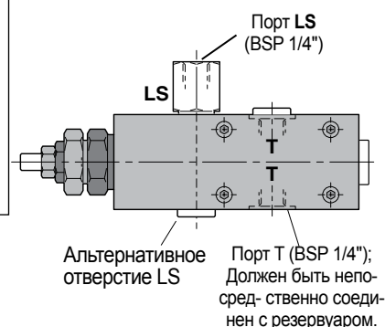
Порты регулирующего клапана VP1-095/-110/130.
