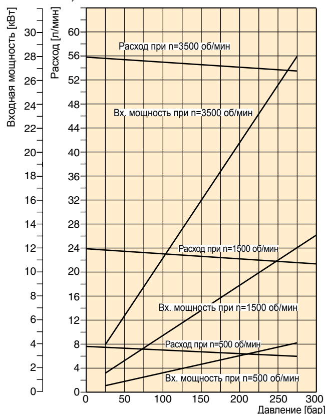
PGP 620 - 41,0 см³/об
