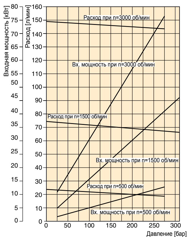
PGP640 - 50,0 см³/об
