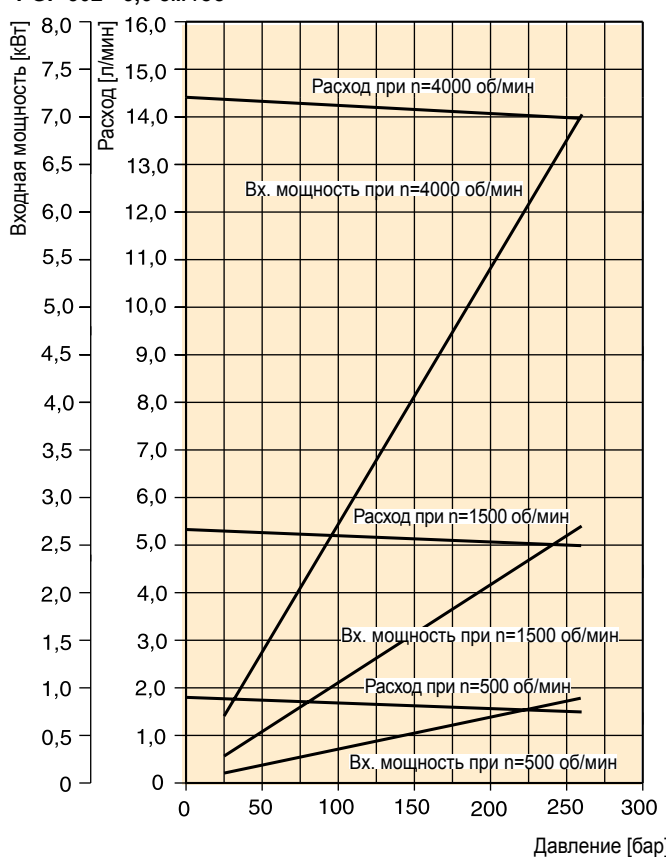
PGP 502 - 3,6 см³/об
