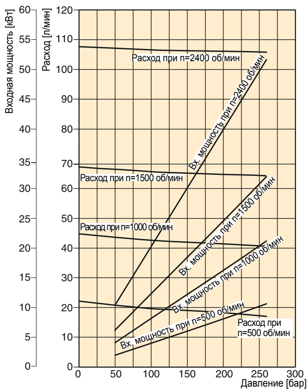
PGP 625 - 45,0 см³/об
