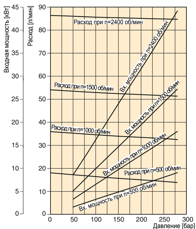
PGP 625 - 45,0 см³/об
