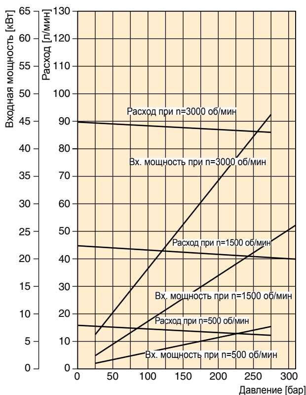
PGP640 - 30,0 см³/об
